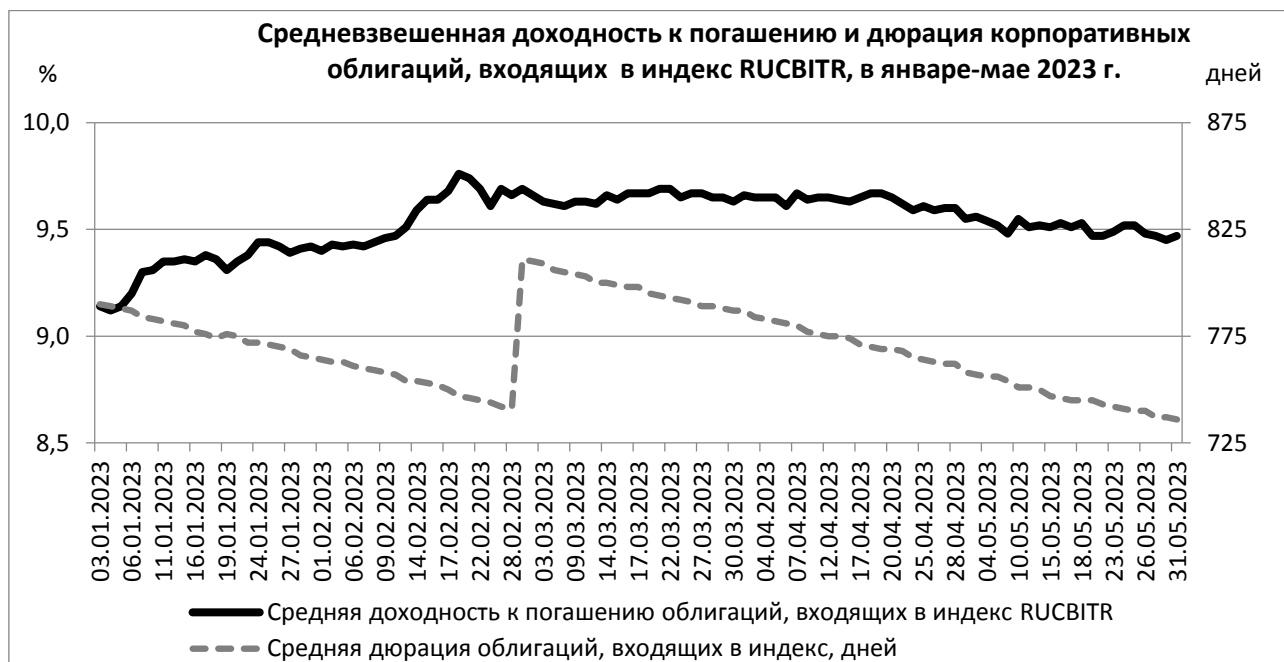
Рисунок 6. Средняя доходность к погашению и дюрация облигаций, входящих в индекс RUCBITR
